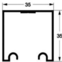
TRILHO STANLEY 35x35 0,460 Kg/m
