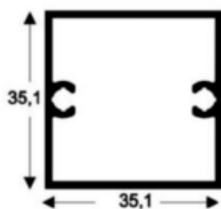
TUBO D 081 0,607 Kg/m
