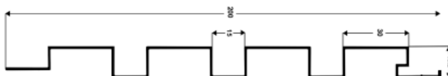
Lambril Ripado 200 mm 1,035 Kg/m
