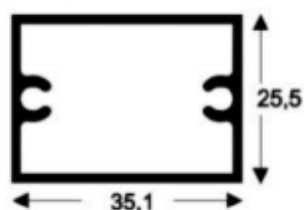
TUBO D 055 0,504 Kg/m
