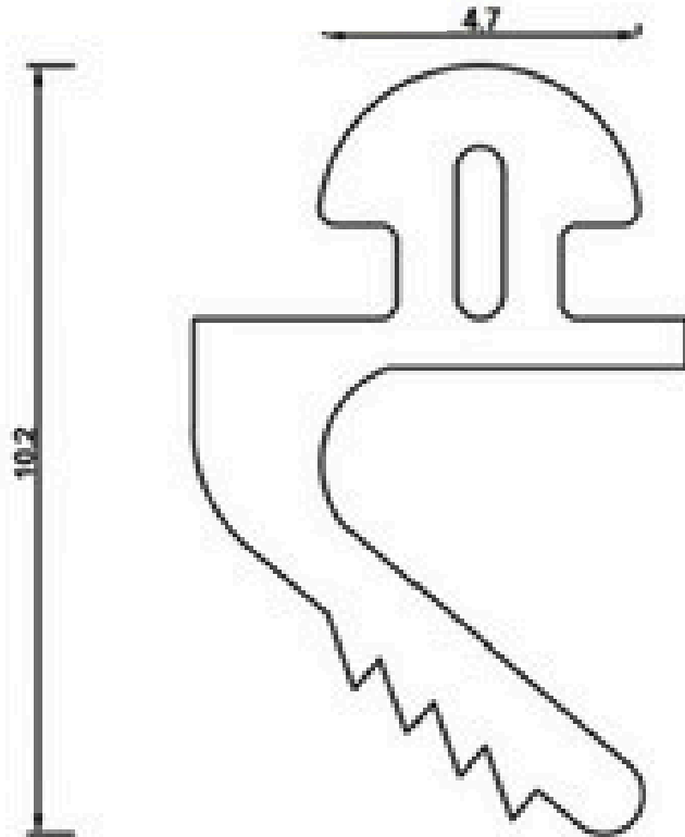
BORRACHA EPDM GUA 239
