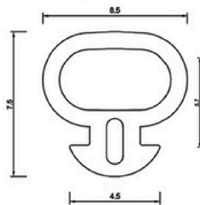
BORRACHA EPDM FAA 202
