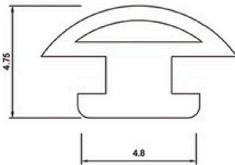
BORRACHA EPDM GUA 053
